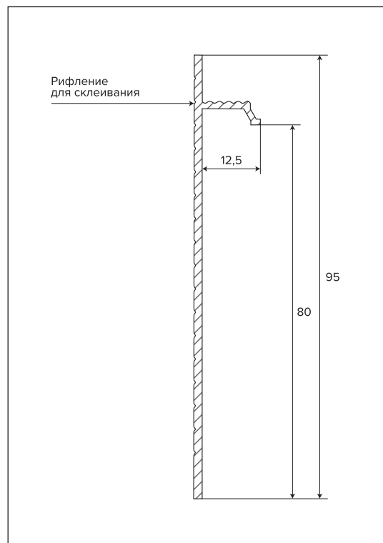
Сечение потайного плинтуса, 95 мм
