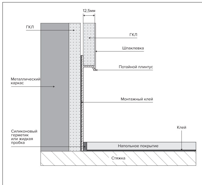
Пример монтажа. Вертикальный разрез
